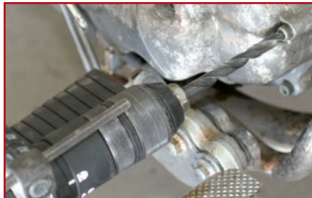
7. Abbohren des defekten Schraubenkopfes
