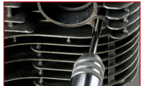
11. ... Gewinde für Helicoil-Reparatur-Einsatz schneiden ...
